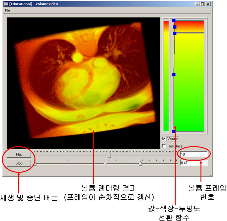
그림 2. 시간의 변화에 따라 심장이 뛰는 모습을 스캔하여 얻어진 시변 볼륨 데이터를 대화형 볼륨 비디오 플레이어로 실행한 예제.
