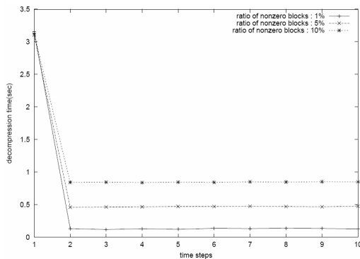
그림 9 압축된 바다 온도 데이터 각 프레임의 압축 해제 시간. 압축 변수값 \tau = 5\% , \lambda = 1\%, 5\%, 10\% .
