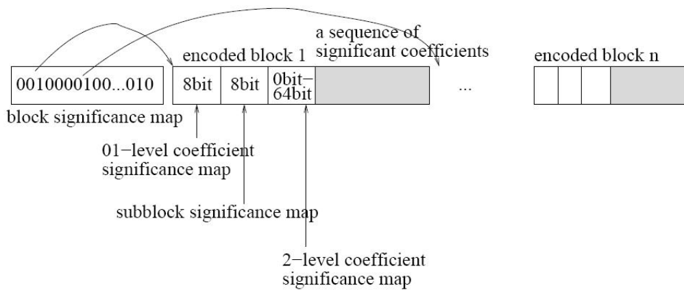
그림 4. 빠른 압축 해제 속도와 높은 압축률을 지원하는 인코딩 방법
