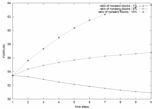
그림 8 압축된 바다 온도 데이터 각 프레임의 PSNR. 압축 변수값 \tau = 5\% , \lambda = 1\%, 5\%, 10\% .
