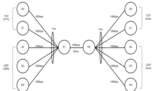
그림 3. ns-시뮬레이션 네트워크 Fig. 3 Network configuration for ns simulations
