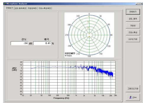
그림 5. B&K 4133 측정 결과
