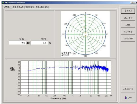
그림 6. OK-801 측정결과 Fig. 6. A measurement results of OK-801 microphone
