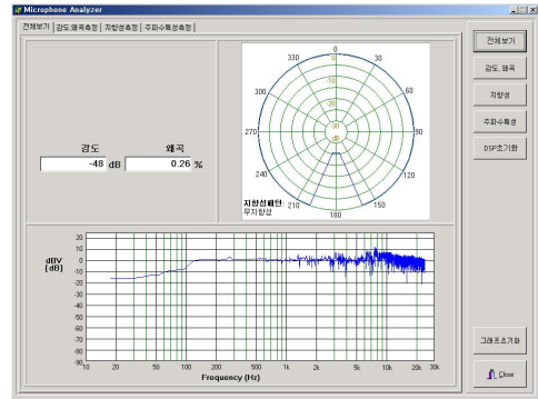
그림 8. N/D 857K 측정결과 Fig. 8. A measurement results of N/D 857K microphone
