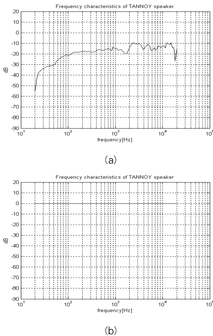
그림 2. 표준 스피커의 주파수 응답특성 및 보정된 스피커의 주파수 응답특성
