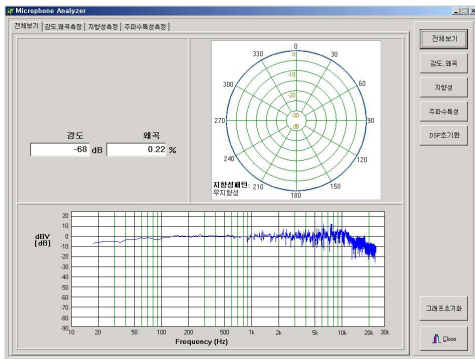
그림 7. ECM-101 측정결과 Fig. 7. A measurement results of ECM-101 microphone
