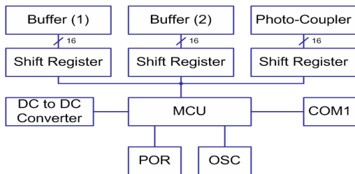
그림 4. 모니터링 보드의 구성 Fig. 4 Monitoring Board Configuration
