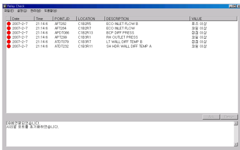
그림 14. 복합적인 에러의 경우 감시 프로그램 Fig. 14 Monitoring Program of Mixed Error Status
