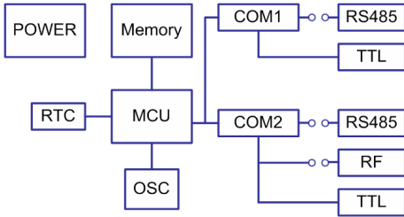
그림 6. 마스터 보드의 구성 Fig. 6 Master Board configuration
