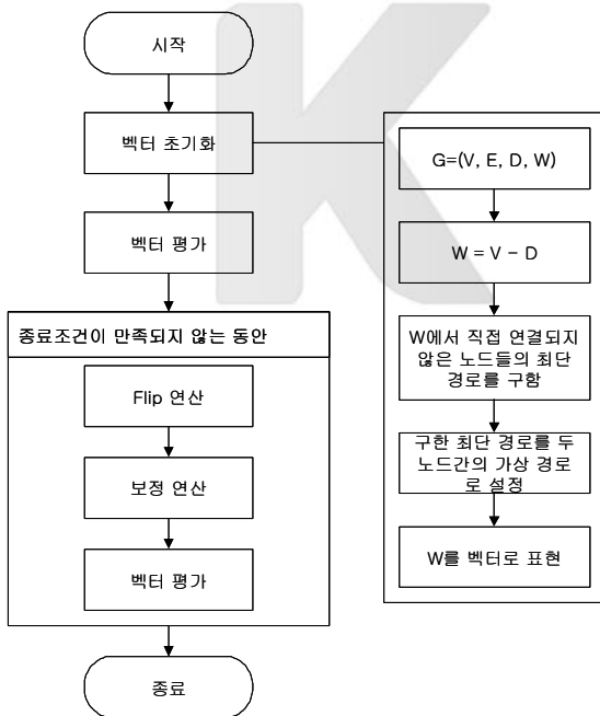
그림 5. 제안된 SA 알고리즘 Fig 5. Proposed SA Algorithm
