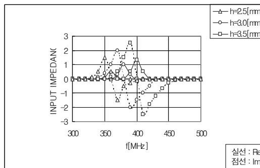
그림 4. 개루우프 높이 변화에 따른 공진주파수와 임피던스 변화 특성 Fig. 4 Resonance frequency and impedance variation characteristics via varying of the loop height
