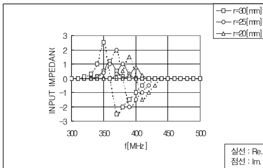
그림 2. 개루우프 반경 변화에 따른 공진주파수와 임피던스 변화 특성 Fig. 2 Resonance frequency and impedance variation characteristics via varying of the loop radius
