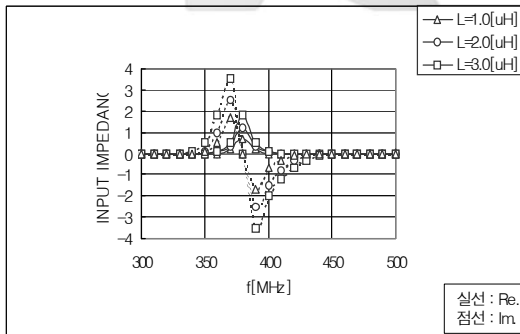
(b) L=1.0, 2.0, 3.0[uH] 경우
