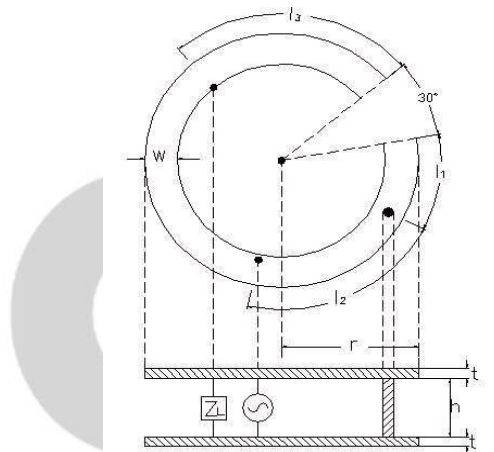
그림1. 해석 안테나 모델 Fig.1 Analysed antenna model
