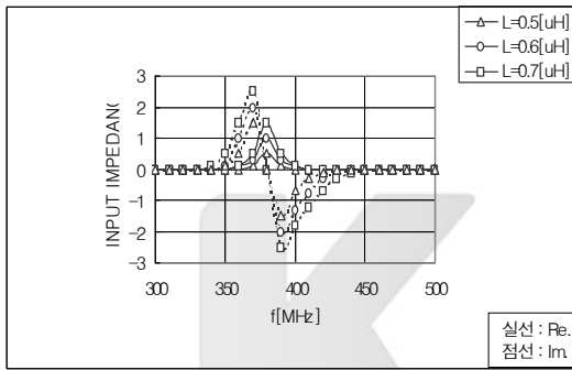
(a) L=0.5, 0.6, 0.7[uH] 경우
