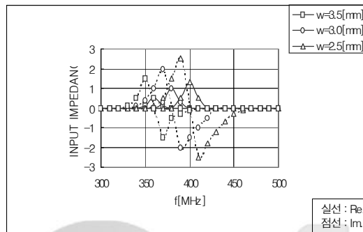
그림 3. 개루우프 선로 폭의 변화에 따른 공진주파수와 임피던스 변화 특성 Fig. 3 Resonance frequency and impedance variation characteristics via varying of the wire width
