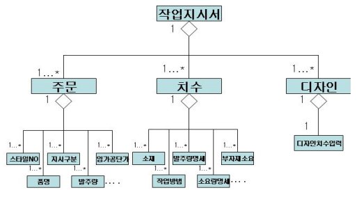
그림 8. WorkSheet데이터베이스의 세부항목 다이어그램 Fig. 8 Details item Diagram of WorkSheet Database
