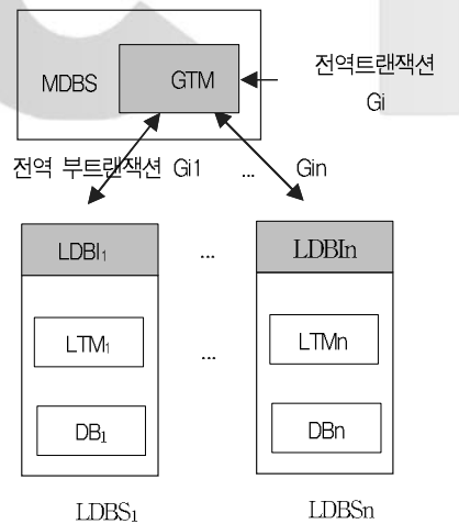
LDBI : 지역 데이터베이스 연계부 (Local Database Interface) GTM/LTM : 전역/지역 트랜잭션 관리기
