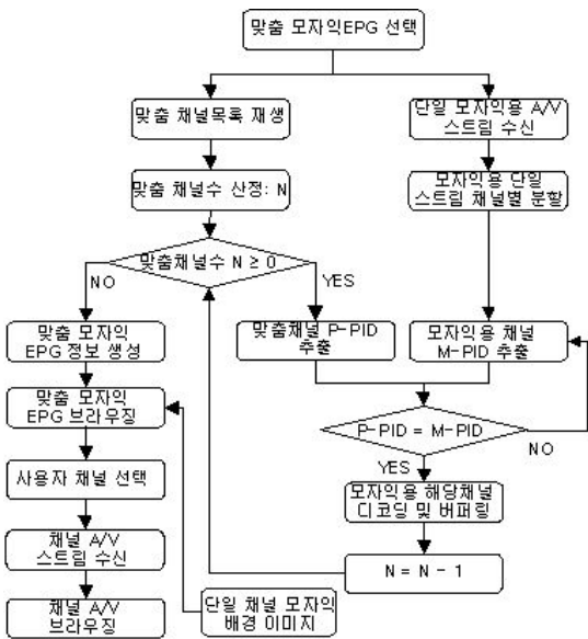
그림 8 가입자단의 맞춤형 모자의 EPG 생성과정 Fig. 8 Generating process of personalized mosaic EPG in Subscriber part
