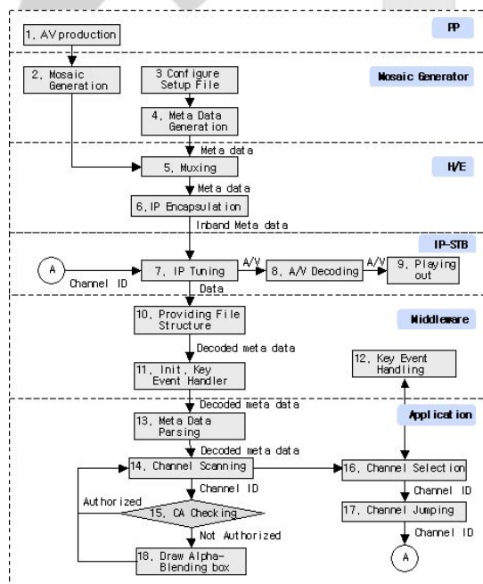
그림 2. IP 기반 고정형 모자이크 EPG 동작과정 Fig. 2 Execution process of fixed mosaic EPG based IP
