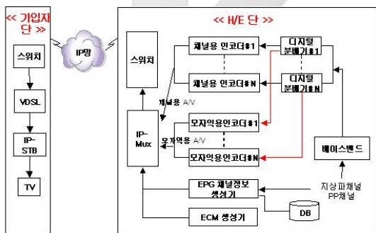
그림 4. 맞춤형 동영상 모자의 EPG 서비스 모델 Fig. 4 Service model for personalized AV mosaic EPG
