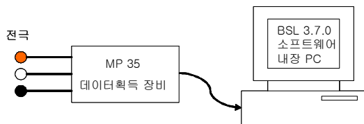
그림 1. 뇌파 측정 시스템 Fig. 1 EEG measurement systems
