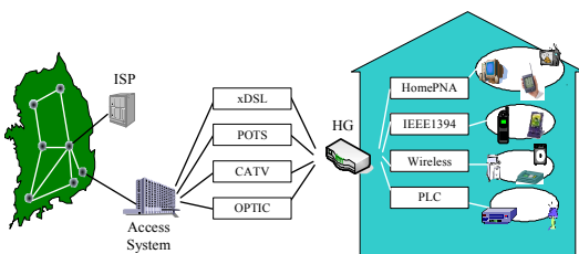
그림 1. 백본/액세스/홈 네트워크 구성 Fig. 1. Configuration of Backbone/Access/Home Network
