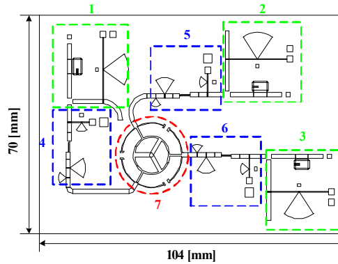
그림 9. 전체 레이아웃 Fig. 9. Final Layout
