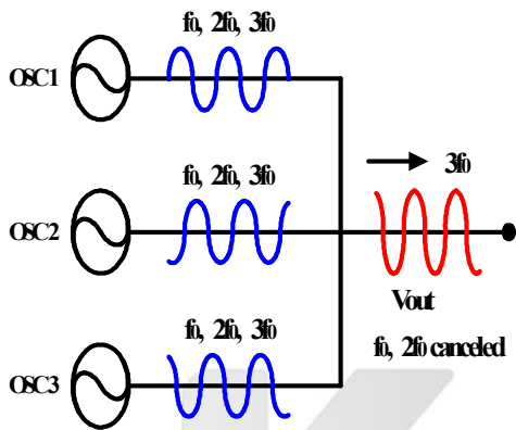
그림 2. Triple-push 발진기 구조 Fig. 2. Structure of Triple-push Oscillator
