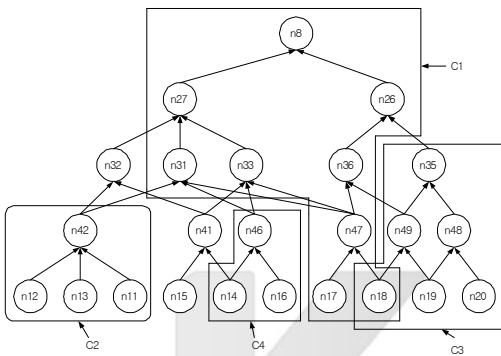
(d) 노드 분할 사용하여 생성된 매핑 가능 클러스터 C2, C3, C4 (d) Feasible cluster generation C2, C3, C4 using node separation algorithm
