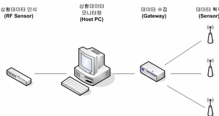
그림 8. 모니터링 시스템 구조 Fig. 8. Monitoring System Architecture
