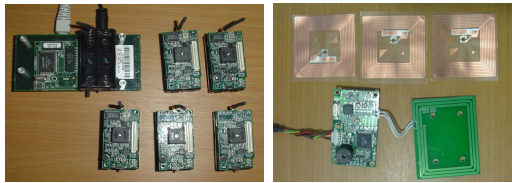
그림 9. 상황정보 수집 센서 Fig. 9. Crossbow Mica Mote, STS 500
