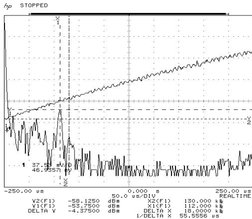
그림 10. 수신 IF 출력단의 측정 결과 Fig 10. Test result of IF output
