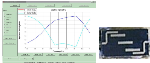
(1) 시뮬레이션 결과 (2) 제작된 필터 그림 4. 설계된 필터 Fig 4. Designed filter
