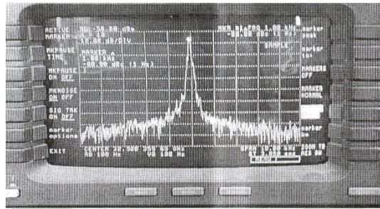
그림 9. VCO의 위상잡음 Fig 9. Phase noise of VCO
