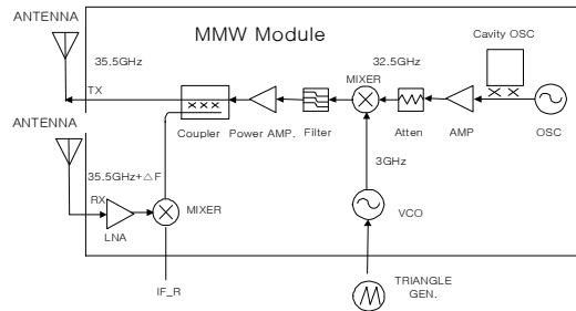
그림 1. 모듈의 블록도 Fig 1. Block diagram of transceiver module
