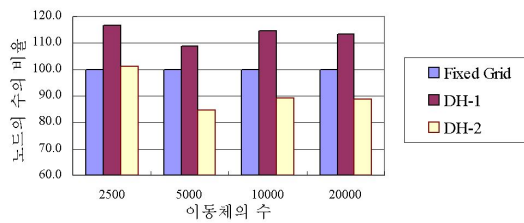
그림 11. 색인 저장 공간의 비교 Fig. 11. A comparison of space utilization.
