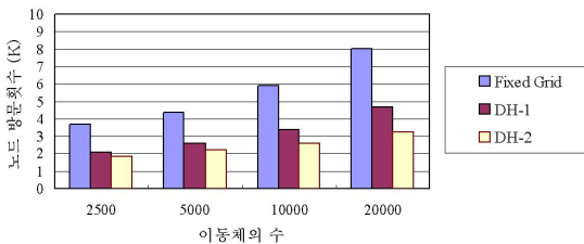
그림 14. 5% 영역 질의 성능 비교 Fig. 13. Performance evaluation for processing 5% range queries in each dimension
