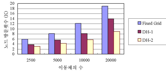
그림 15. 10% 영역 질의 성능 비교 Fig. 15. Performance evaluation for processing 10% range queries in each dimension
