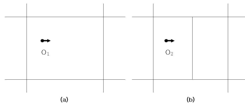
그림 7. 셀의 크기와 색인의 변경의 관계. (a) 그리드 셀 내에서의 이동, (b) 1/2크기로 분할된 셀 내에서의 이동. Fig. 7. The relationship between the size of a cell and updating index. (a) The movement in a grid cell, (b) The movement in a half-size cell.
