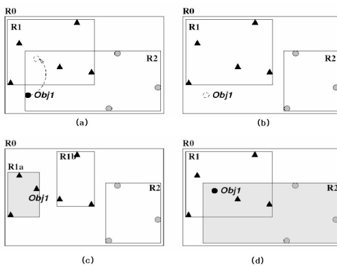
그림 4. R-tree에서의 기존 갱신 방법과 Lazy 갱신 방법의 예. (a) 위치 이동, (b) 기존 방법: Obj1 삭제, (c) 기존 방법: Obj1 삽입과 노드 분할 (d) Lazy 갱신: R2의 MBB 확장 Fig. 4. Example of traditional update algorithm and lazy update algorithm. (a) a movement of the position, (b) traditional update: delete Obj1, (c) traditional update: insert Obj1 and split the node, (d) Lazy update: expand the MBB of R2
