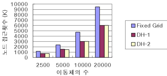
그림 13. 색인 변경을 위한 노드 접근 횟수 Fig. 13. The number of node accesses for updating indexes
