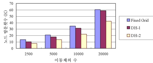
그림 16. 20% 영역 질의 성능 비교 Fig. 16. Performance evaluation for processing 20% range queries in each dimension
