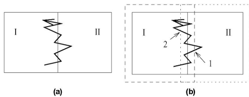
그림 2. Zigzag 문제. (a) 셀 경계를 이동하는 이동체, (b) 중첩된 확장 MBR들 Fig. 2. Zigzag problem. (a) an moving object along the border, (b) overlaped expansion MBRs
