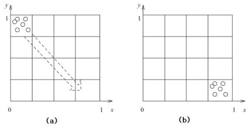
그림 3. 이동체의 비대칭 분포. (a) 시각 t0에서의 이동체들, (b) 시각 t1에서의 이동체들 Fig. 3. Skewed distribution of objects. (a) moving objects at t0, (b) moving objects at t1
