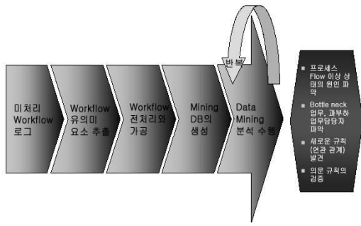
그림 2. 마이닝을 이용한 워크플로우 로그 분석 수행 단계 Fig 2. Workflow Log Analysis Execute Phase Mining
