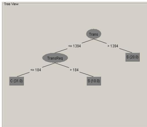
그림 5. 비즈니스 프로세스 분석 결과(의사결정나무) Fig. 5. Business process analysis result(Decision Tree)
