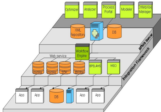
그림 1. BPMS 아키텍처 Fig 1. BPMS Architecture
