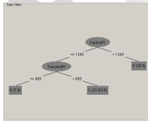
그림 6. 비즈니스 프로세스 분석 결과(Decision Tree) Fig. 6. Business process analysis result(Decision Tree)
