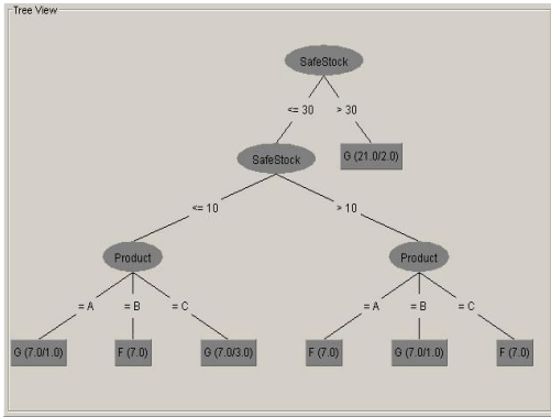
그림 8. 비즈니스 프로세스 분석 결과(Decision Tree) Fig. 8. Business process analysis result(Decision Tree)
