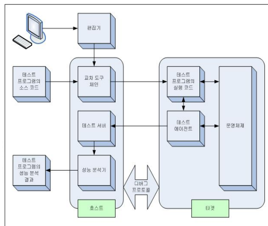
그림 1. 임베디드 소프트웨어의 교차 개발 환경 Fig 1. Cross-Development Environment in Developing Embedded Software
