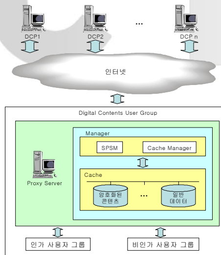
그림 2 시스템의 구성 Fig 2. Configuration of systems
