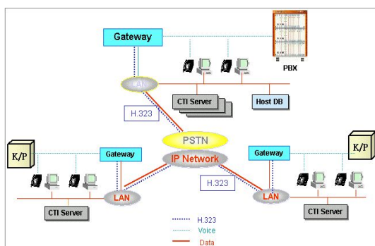
그림 1. VoIP 서비스 망 Fig. 1 VoIP Service Network
