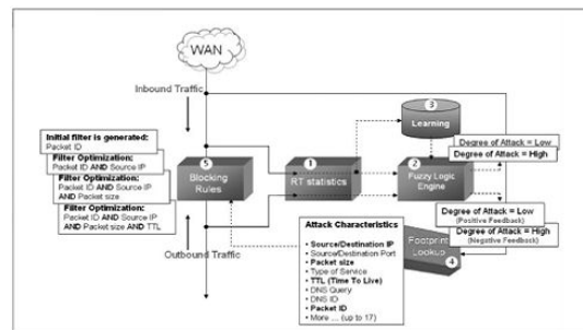
그림 13. 패킷의 RT 통계를 통한 트래픽 양을 측정 Fig. 13 Measure Miss traffic through RT statistics of a packet.
