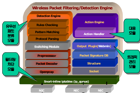
그림 3.2 트래픽 침입탐지/차단 엔진 구조 Fig. 3.2 W-Sensor/TMS Engine Structure
