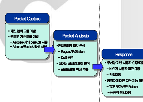
그림 3.4 W-Sensor 시스템 구조 Fig. 3.4 W-Sensor System Structure
