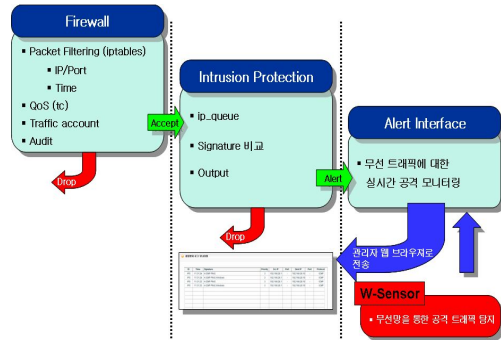
그림 3.8 W-TMS의 구조 Fig. 3.8 W-TMS Structure
