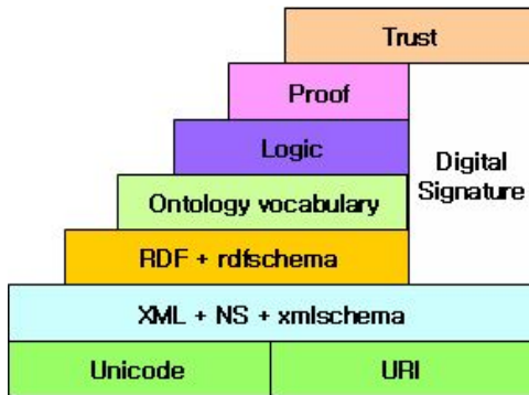
그림 1. 시맨틱 웹의 구조 Fig 1. Structure of the Semantic Web
