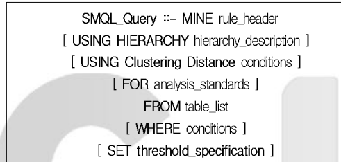
그림 9. 공간 특성화 질의어의 BNF Fig. 9 BNF of spatial characterization query
