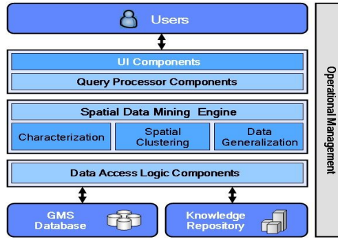
그림 8 공간 특성화 시스템 Fig.8 Spatial Characterization System
