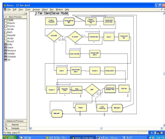
그림 5. 2-계층 C/S 시뮬레이션 모델 Fig. 5. 2-tier C/S Simulation Model
