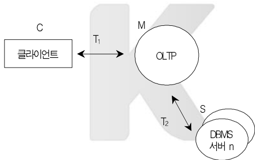
그림 2 3-계층 C/S 구성도 Fig. 2 3-tier C/S Structure
