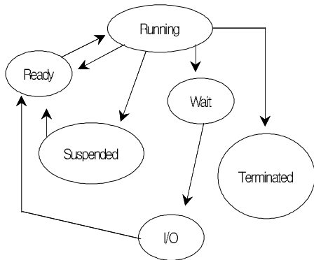
그림 4. 프로세스 상태 전이도 Fig. 4 Process State-Transition Diagram
