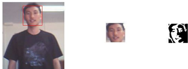
그림 11. 피부색 참조 맵을 이용하여 생성한 이진 영상 Fig 11. Binary image using the Skin color map
