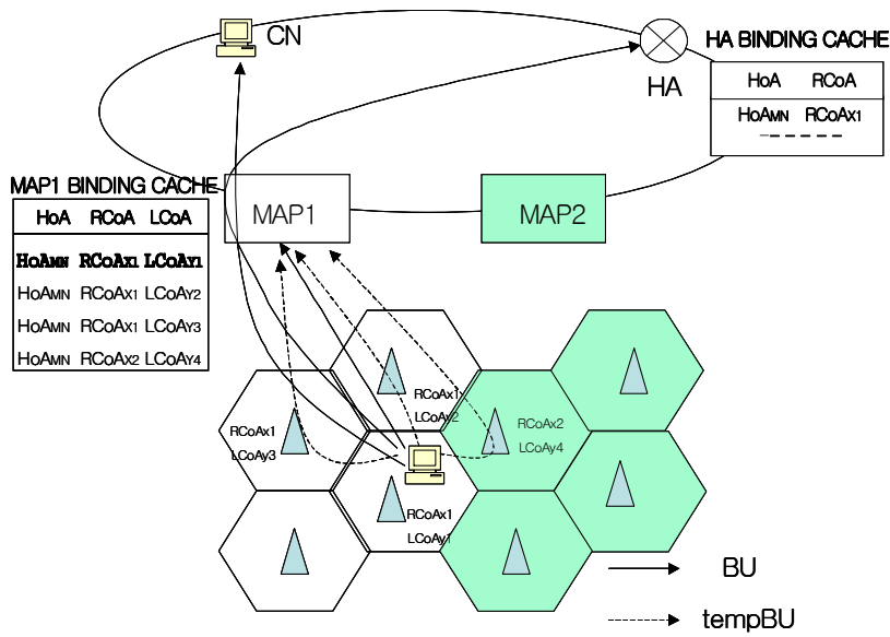
그림 1. 핸드오프 지원을 위한 제안된 멀티캐스트 기법 Figure 1. Proposed Multicast scheme for supporting handoff
