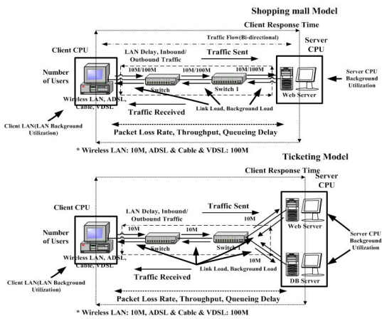
그림 2. LAN의 QoS 측정망 모형 Fig. 2 QoS of LAN Measurement Model
