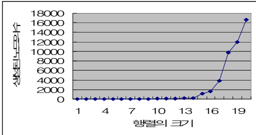
그림 4. 행렬의 크기에 따른 travel_A가 생성하는 노드의 수의 변화 Figure 4. Number of generated nodes vs. matrix sizes
