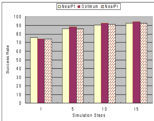
그림 6. 정규화 방법에서 실험 단계에 따른 검색 성공률 Fig 6. Success rates at the simulation steps in regular methods
