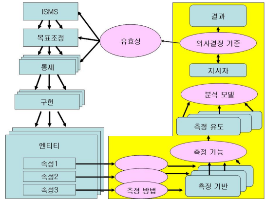
그림 4 정보보안 일반측정 모형 Fig 4. Information security general measurement model
