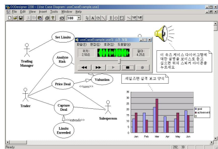
그림 7 음성을 이용한 문서화의 예 Fig. 7 Screen shot of OODesigner Embedding voice objects
