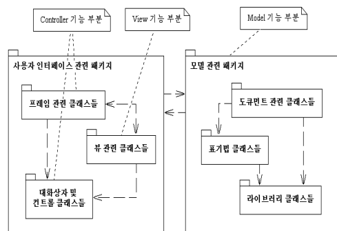
그림 1 OODesigner의 시스템 개략 설계 Fig. 1 Overall Design of OODesigner
