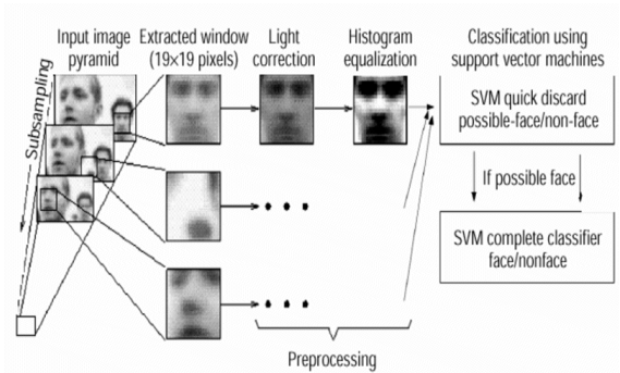
그림 9 SVM을 이용한 얼굴 검색 알고리즘 Fig9. Face retrieval system using SVM
