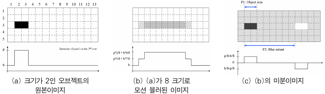
그림 1. 오브젝트가 블러의 크기보다 작은 경우 Fig. 1 Case when the blur extent is larger than the size of the object
