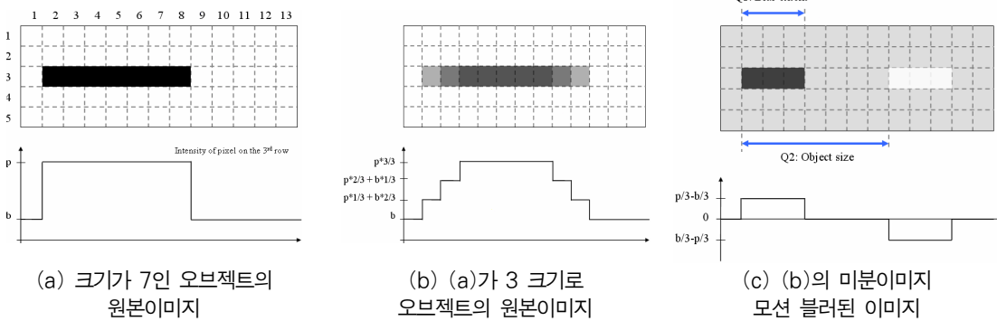
그림 2. 오브젝트가 블러의 크기보다 큰 경우 Fig. 2 Case when the blur extent is smaller than the size of the object
