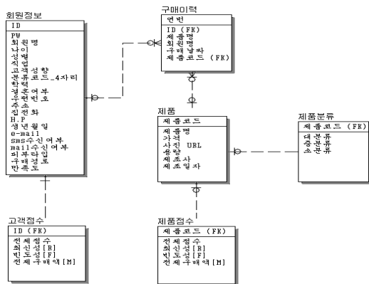
그림 2. ERD로 나타낸 데이터베이스 구조 Fig. 2. ERD of database structure
