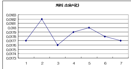
그림 6. 추천조건별 전체 건수별 추천 처리 시간 결과 Fig. 6. The result of processing time of total count for recommendation each condition type (unit: sec)
