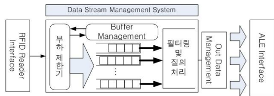
그림 3. 제안 모델 Fig. 3 Proposal Model
