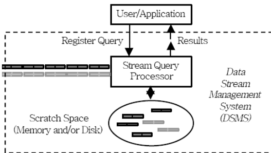
그림 2. 데이터 스트림 관리 시스템 Fig. 2 Data Stream Management System(DSMS)
