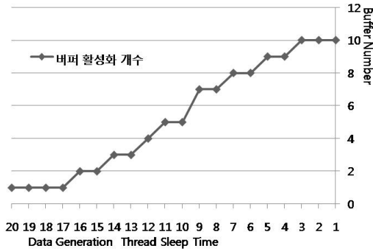
그림 6. 데이터 유입량에 따른 동적 버퍼 증감 수 Fig. 6 The changes of the dynamic buffer according to the data inflow
