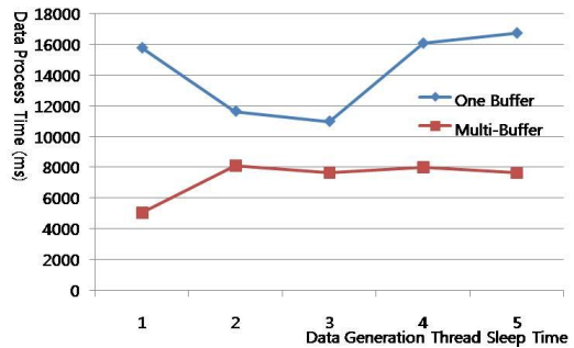
그림 7. 단일 버퍼와 다중 버퍼 데이터 처리 시간 비교 Fig. 7 The comparison of the data processing rates of the single and multiple buffers
