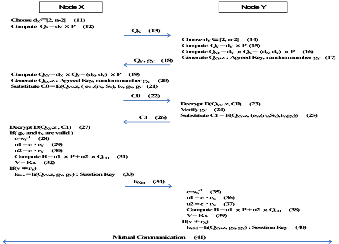
그림 4. 노드간 상호 인증 절차 Fig 4. Mutual Authentication Process between Nodes
