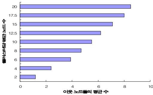
그림 6. 네트워크 밀집도에 따른 클러스터 노드의 평균 수 Fig. 6. A Number of Cluster Node in Network Density
