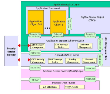
그림 4. ZigBee 스택 구조 Fig 4. ZigBee Stack Architecture
