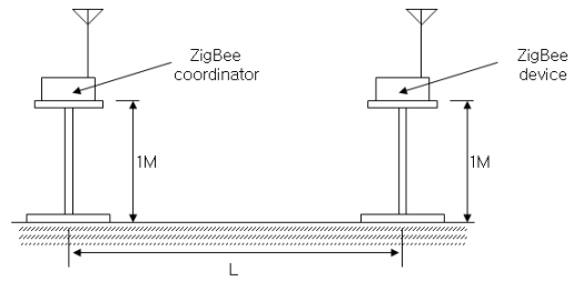
그림 5. LOS(Line of Sight) 환경에서의 통신거리 측정 Fig 5. Estimation of Communication Distance in LOS Environments
