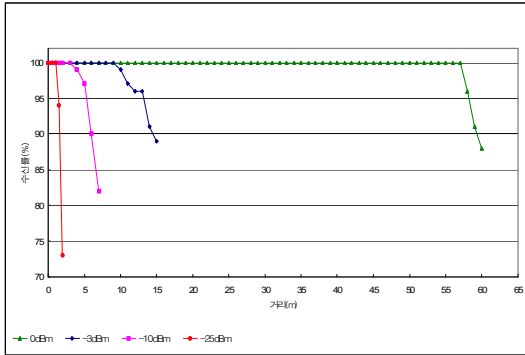
그림 7. 출력에 따른 ZigBee 모듈의 통신 거리(안테나: 3dBi Chip - 3dBi Chip) Fig 7. Communication Distance of ZigBee Module to Power(Antenna: 3dBi Chip - 3dBi Chip)
