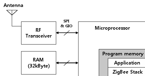
그림 1. 시스템 구조 Fig 1. System Architecture
