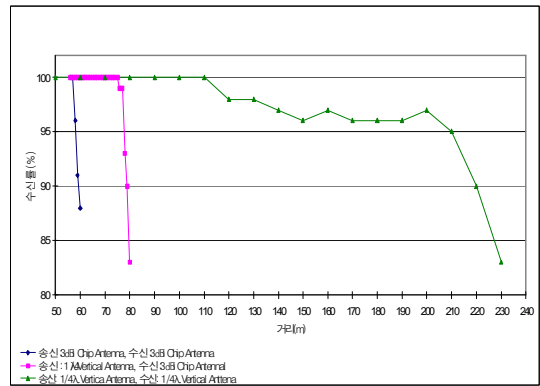
그림 6. 안테나에 따른 ZigBee 모듈의 통신 거리(출력: 0dBm 기준) Fig 6. Communication Distance of ZigBee Module to Antennas(Power: 0dBm)
