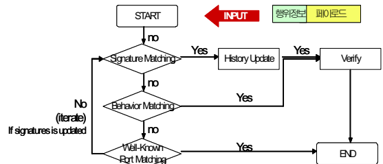
그림 4. 통합 기반의 방법론(8) Fig 4. Hybrid-based Identification Method(8)
