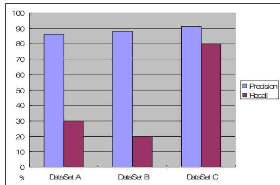
그림 8. 제안 방식의 결과 Fig 8. Result of Proposed Method
