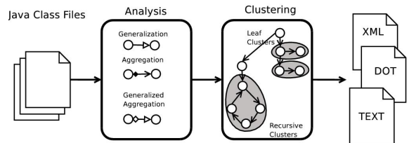
그림 1. 시스템의 개요 Fig 1. Overview of System
