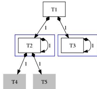
그림 18. 그림 17의 클래스 구조와 관련성 Fig. 18. Classes and Relationship of Fig 17
