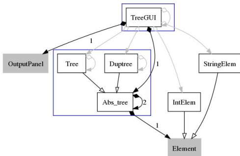
그림 20. TreeGUI 프로그램의 구조와 관련성 Fig 20. Resulting Graph of TreeGUI Program
