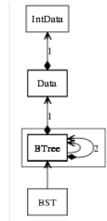
그림 21. 변형된 이진 검색 트리 프로그램 Fig 21. Modified Binary Search Tree Program
