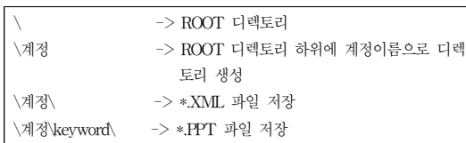
그림 10. 서버에 존재하는 콘텐츠 관리를 위한 디렉터리 구조 Fig 10. Directory structure for contents management that exist on server
