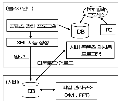
그림 1. 전체 시스템 구성도 Fig 1. Total system architecture
