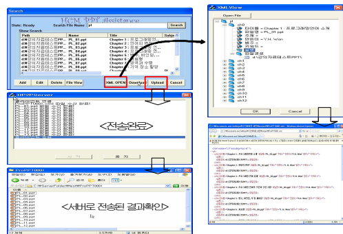
그림 18. XML과 콘텐츠들을 서버로 전송한 결과 Fig 18. Result that transmits XML and contents to server
