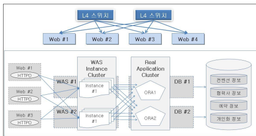
그림 5. WAS를 이용한 3-tier구조 Fig. 5. The 3-tier structure that used WAS.
