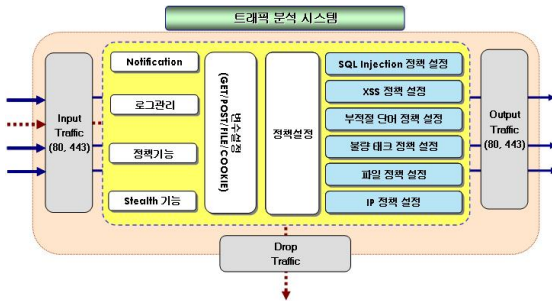
그림 3. 트래픽 분석 시스템 Fig 3. Traffic Analysis System
