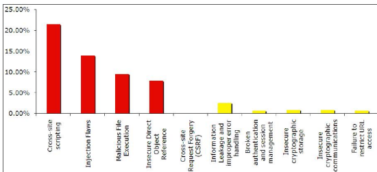
그림 2. MITRE 취약점 경향 (2006) Fig 2. MITRE Vulnerability Trends for 2006
