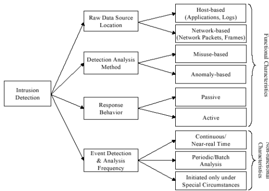
그림 1. IDS의 구조 Fig 1. IDS Framework (ISO/IEC TR 15947)
