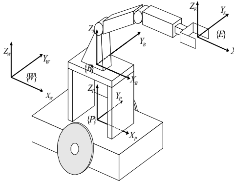
그림 2. 이동매니퓰레이터의 기구학 해석 Fig. 2. Kinematic analysis of the mobile manipulator
