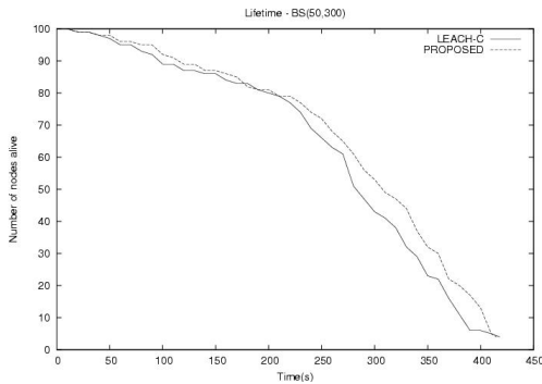
Fig 7. Lifetime considering the position (50,300) of BS 그림 7. BS(50,300)일 경우의 라이프타임
