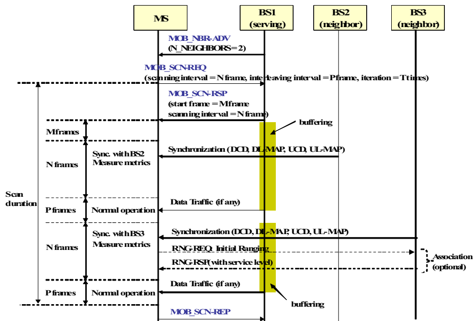
그림 2. IEEE 802.16e 표준에서 정의된 스캔 프로세스.
