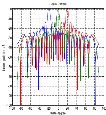
그림 2. 제안 알고리즘 빔 패턴 (dB) Fig 2. Beam pattern of proposed algorithm (dB)
