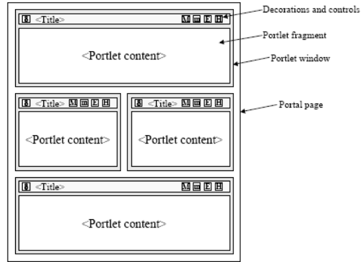
그림 1. 포탈 페이지를 구성하는 포틀릿 Fig 1. Portlets on a Portal Page
