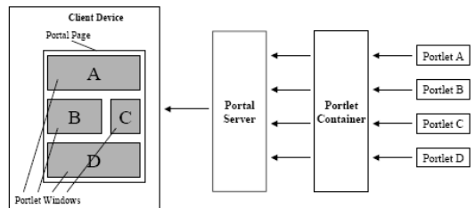
그림 2. 포탈 페이지 생성 과정 Fig 2. Portal Page Creation
