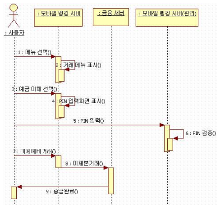
그림 6. 시퀀스 다이어그램 Fig 6. Sequence Diagram
