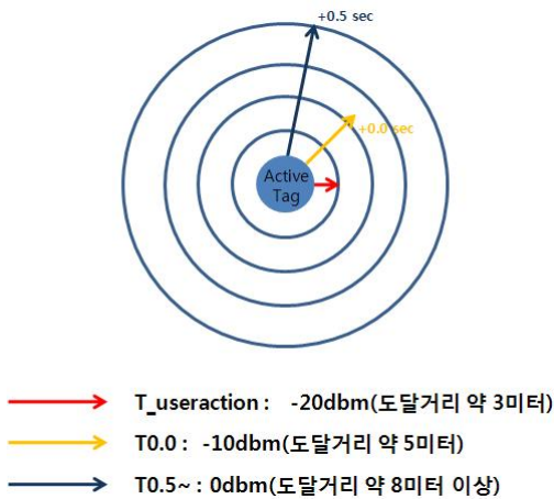
그림 2. 2.45GHz 능동형 태그 Fig. 2. 2.45GHz active tag
