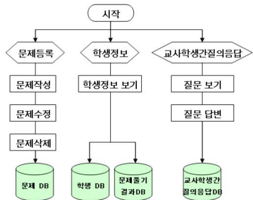
그림 2. 교사모드의 메뉴 및 DB Fig. 2. Instructor menu and DB
